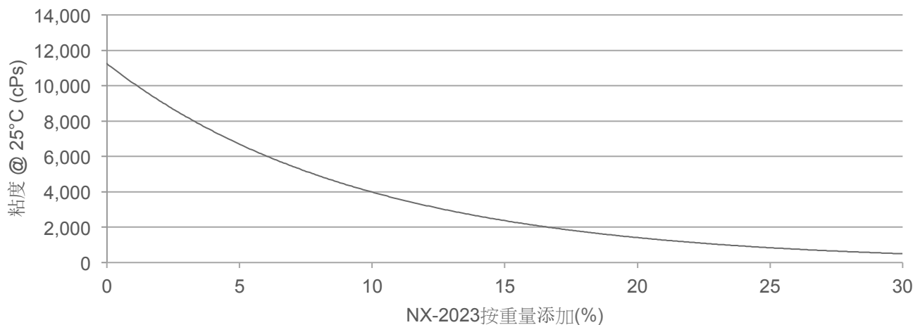
NX-2023与液体环氧树脂混合的稀释曲线图（环氧当量=190）
