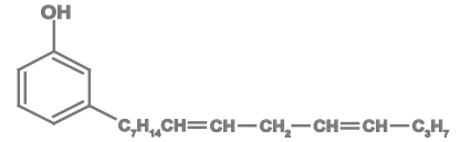
化学结构
